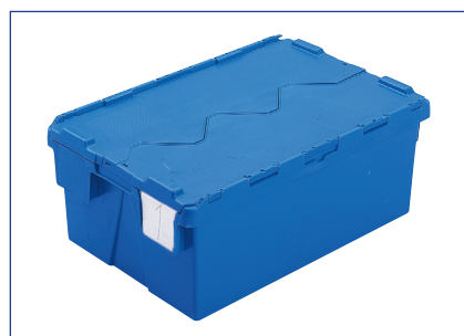
AT642604 - 48 Lit. ext. 600 x 400 x 264 mm int. 530 x 353 x 240 mm gewicht 3,00 kg
