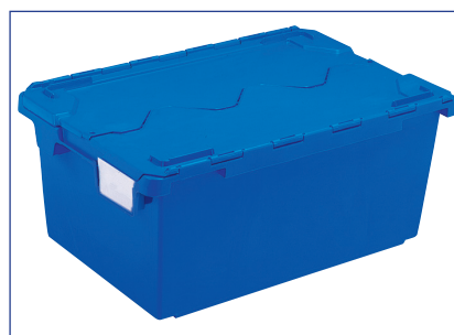
AT704604 - 75 Lit. ext. 714 x 465 x 356 mm int. 598 x 375 x 307 mm gewicht 4,60 kg
