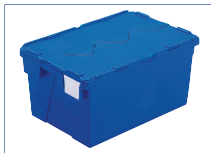
AT644004 - 70 Lit. ext. 600 x 400 x 400 mm int. 521 x 343 x 375 mm gewicht 3,70 kg
