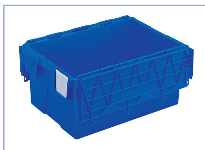
AT643104 - 54 Lit. ext. 600 x 400 x 306 mm int. 514 x 350 x 281 mm poids 3,20 kg
