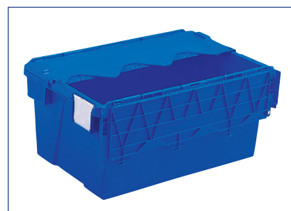
AT643604 - 65 Lit. ext. 600 x 400 x 365 mm int. 508 x 346 x 340 mm poids 3,50 kg
