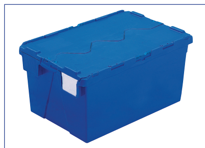
AT644004 - 70 Lit. ext. 600 x 400 x 400 mm int. 521 x 343 x 375 mm poids 3,70 kg
