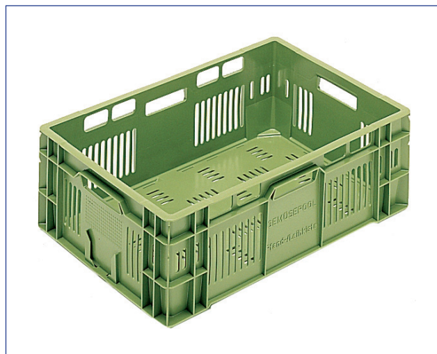
Réf. V-6419 - 38 lit. - 1.710 gr. ext. 600 x 400 x 190 mm int. 565 x 365 x 185 mm
