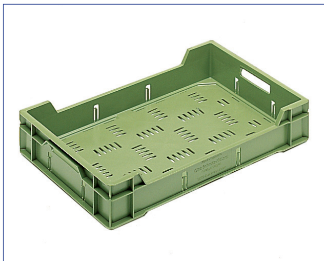
Réf. V-6410-11 - 12 lit. - 1.180 gr. ext. 600 x 400 x 65/110 mm int. 565 x 365 x 60/105 mm
