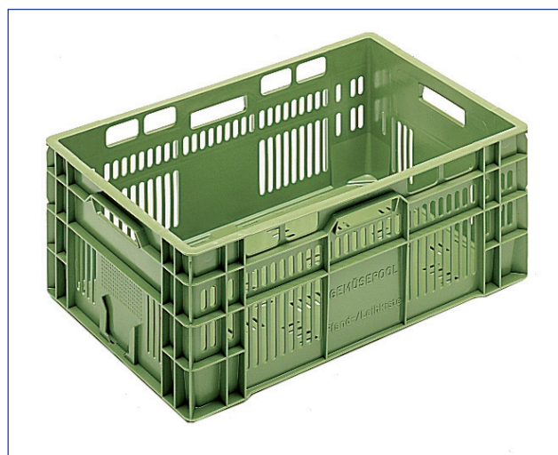
Réf. V-6423 - 46 lit. - 1.980 gr. ext. 600 x 400 x 230 mm int. 565 x 365 x 225 mm
